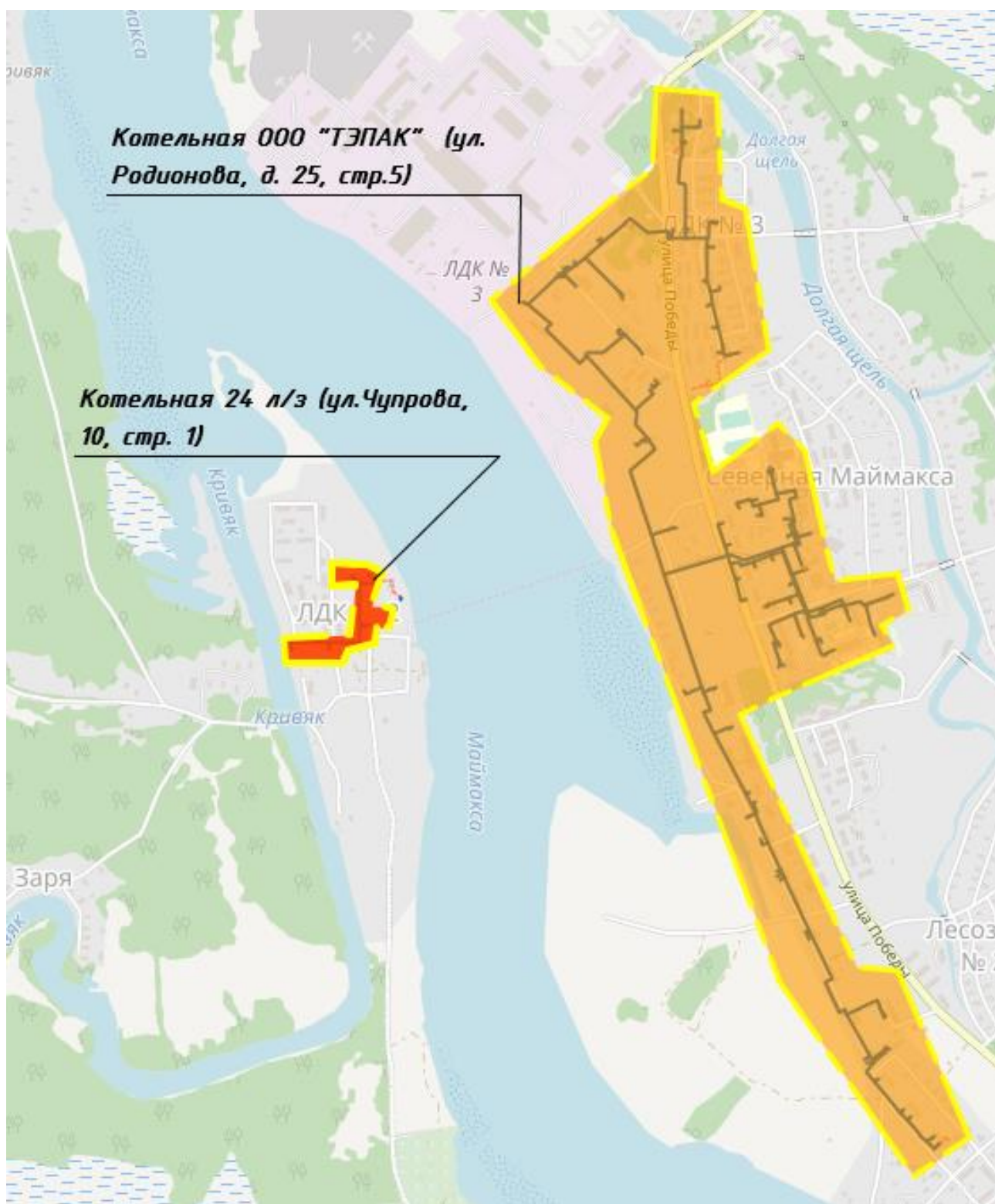
Рисунок 32. Зоны действия котельной ООО «ТЭПАК» ул. Родинова, д. 25, стр. 5 и котельной 24 л/з ул. Чупрова 10, стр. 1
