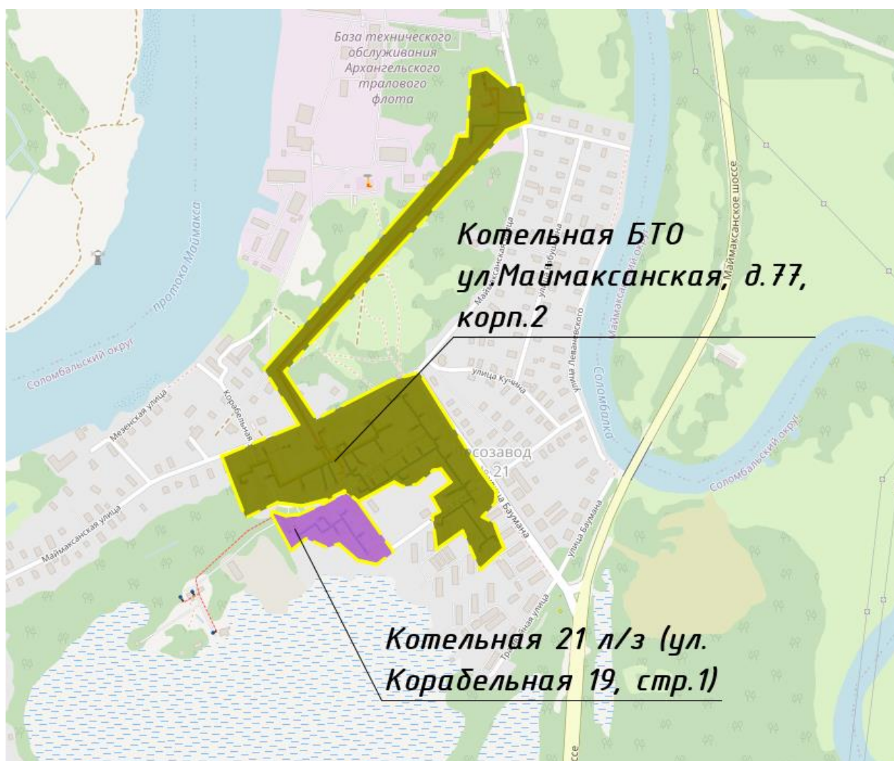
Рисунок 3. Зоны действия котельных БТО ул. Маймаксанская, д. 77, корп. 2 и Котельной 21 л/з ( ул. Корабельная 19, стр.1)
